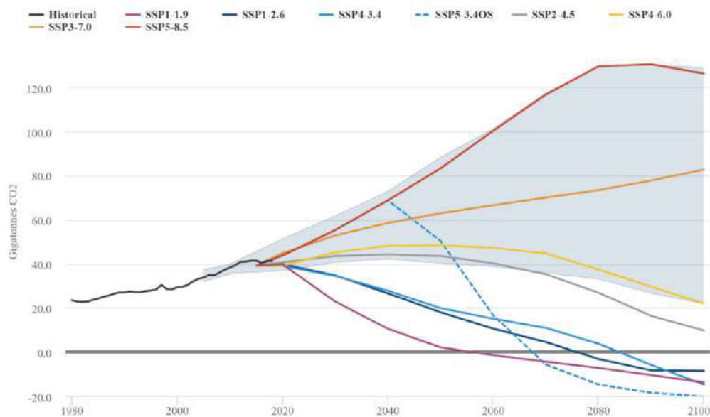
Figura 42 - Scenari futuri delle emissioni di CO2 presenti nel CMIP6, nonché emissioni storiche di CO2 (in nero). L'area ombreggiata rappresenta la gamma di scenari di base senza criteri. Dati dal database SSP (Fonte Carbonbrief.org)
