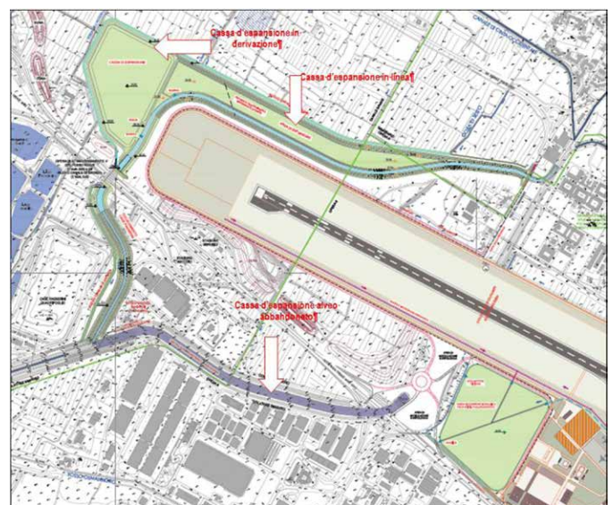
Stralcio planovolumetrico degli interventi di sistemazione idraulica del Fosso Reale
