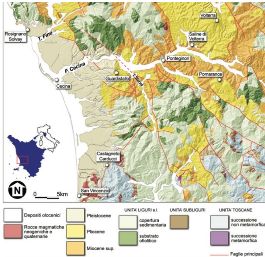
Figura 3 - Schema geologico semplificato dell'area della Val di Cecina (da: Carta Geologica della Toscana, 1:250.000, con modifiche). – Geological sketch map of the study area (from: Geological map of Tuscany, 1:250,000, modified).
