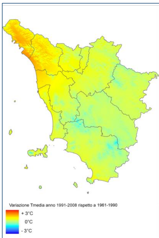
Figura 5 - Mappa delle variazioni di temperatura media annua (°C) del periodo 1991-2008, rispetto al trentennio di riferimento 1961-1990. (Fonte: LaMMA, 2010. Dati: Aeronautica Militare, Centro Funzionale, ARSIA).
