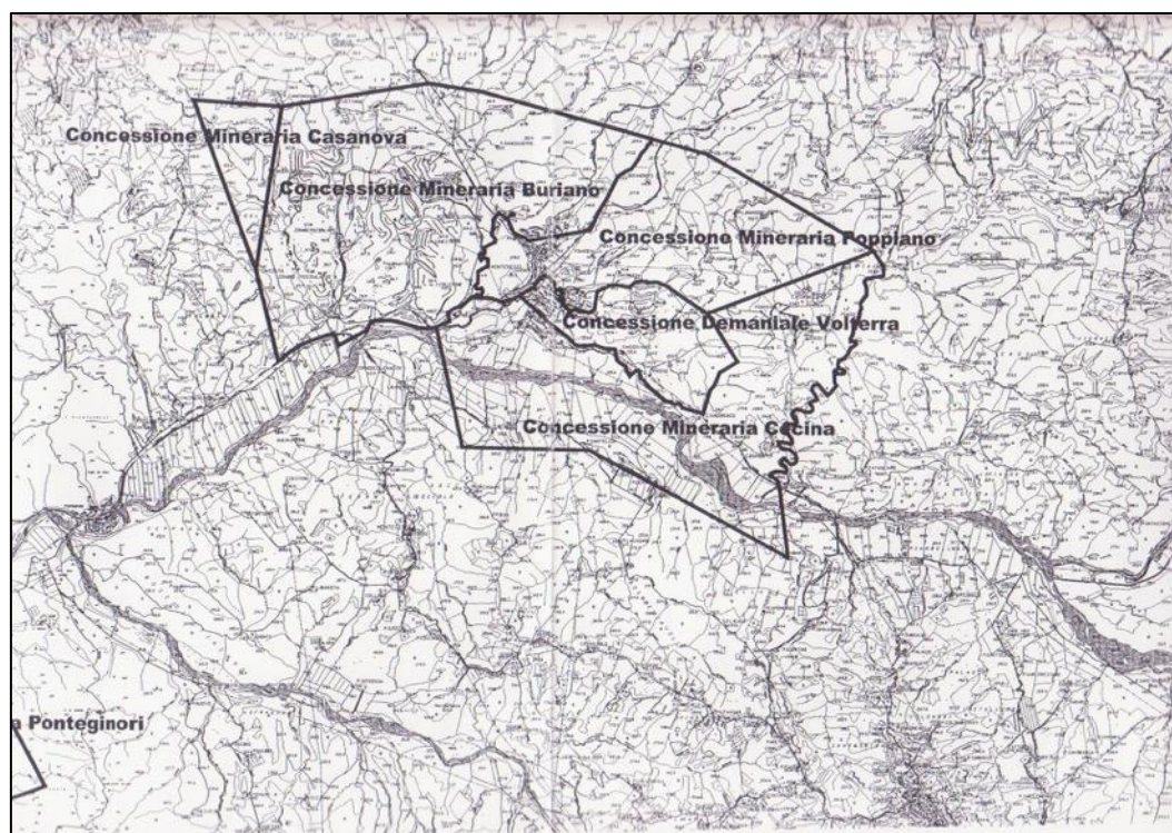
Figura 18 - Concessioni minerarie per l'estrazione del salgemma intorno al paese di Saline di Volterra. Fonte: sito dell'ARPAT
