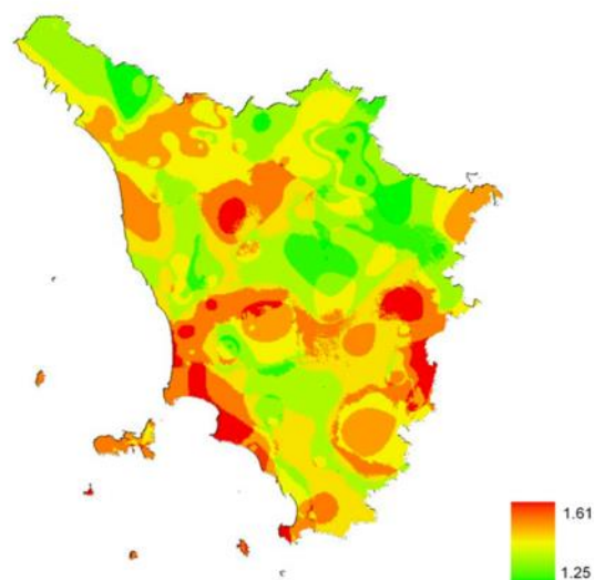
Figura 6 - Mappa di qualità del clima: analisi strutturale e congiunturale di aridità e siccità. (Fonte: LaMMA, 2010)
